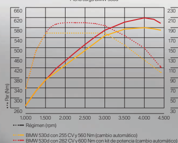
Prestaciones del BMW 530d con el kit de potencia BMW M Performance Plena carga BMW 530d
